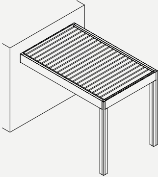
Anclaje a pared invisible Invisible wall anchor
