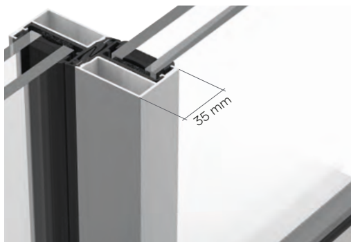
Nudo central reducido de 35 mm Slim interlock of only 35 mm
