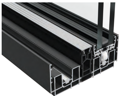
Roulement dans le vantail Configurations de vantaux jusqu'à 600 kg
