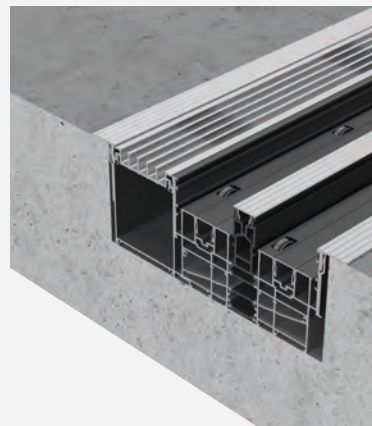
Caniveau de drainage avec grille aluminium
